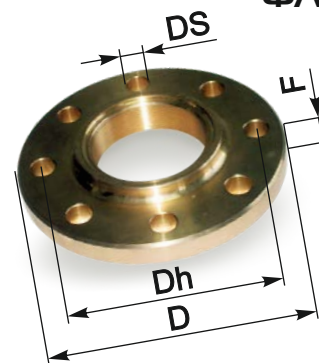
ФЛАНЕЦ
