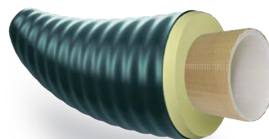
ТВЭЛ-ПЭКС-115-К (с армирующей системой)
