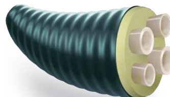
ТВЭЛ-ПЭКС-115-К (с армирующей системой)
